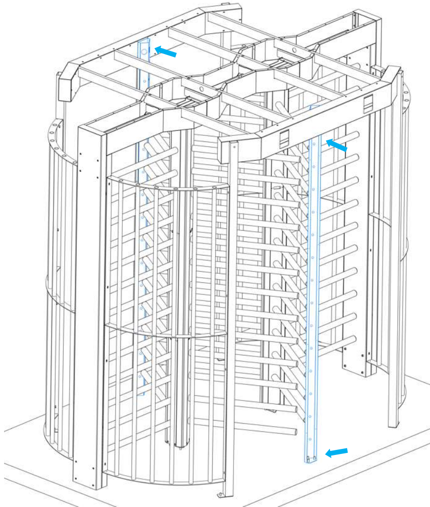
Fijación de la base
