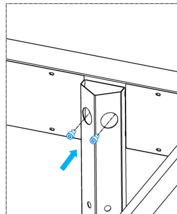
Fijación Base Superior
